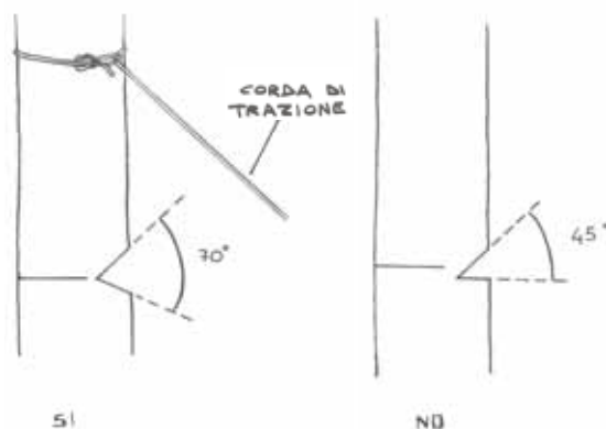
Taglio cimale o toppe in posizione verticale
