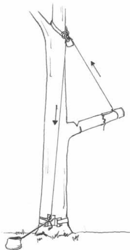
Effetto carrucola in una fase dello smontaggio
